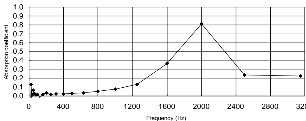
Fig. 6 - Coeficientul de absorbție pentru proba 6 (rășină formaldehidică 20% + cenușă de termocentrală 10%+ deșeu polistiren 70%) / Absorption coefficient for sample 6 (20% formaldehyde resin + 10% power plant ash + 70% polystyrene waste)
