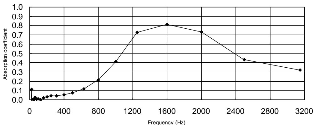
Fig. 4 - Coeficientul de absorbție pentru proba 4 (rășină formaldehidică 20% + deșeu de gunoi 80%) / Absorption coefficient for sample 4 (20% formaldehyde resin + 80% sterile municipal waste).
