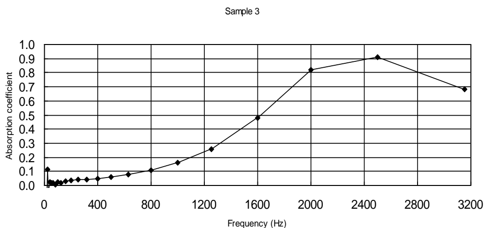
Fig. 3 - Coeficientul de absorbtie pentru proba 3 (rășină formaldehidică 20% + zgură de furnal 80%) / Absorption coefficient for sample 3 (20% formaldehyde resin + 80% furnace slag)
