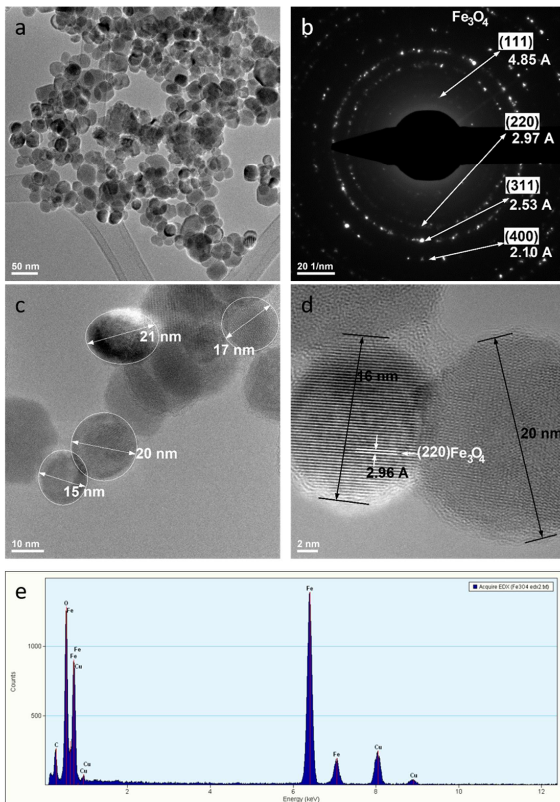
Fig. 3 - TEM of \text{Fe}_3\text{O}_4 : a) BF-TEM image of \text{Fe}_3\text{O}_4 nanoparticles agglomeration; b) selected-area electron diffraction (SAED) pattern for the \text{Fe}_3\text{O}_4 powder associated to the nanoarea in image a; c), d) HR-TEM images; e) EDAX spectrum acquired on the nanoparticles agglomeration from image a. / Rezultate TEM obținute pe nanomaterial \text{Fe}_3\text{O}_4 : a) Imagine BF-TEM a unei aglomerări de nanoparticule; b) imagine de difracție de electroni (SAED) asociată nanoariei din a); c), d) imagini HR-TEM; e) spectru EDAX achiziționat pe aglomerarea de nanoparticule din a).
