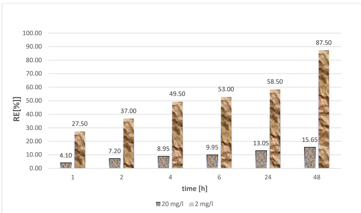
Fig. 5 - The variation of the removal efficiency (RE) % of benzethonium chloride concentration from wastewater versus time (h). Variația eficienței de îndepărtare (RE) % a clorurii de benzetoniu din apa uzată versus timp (h)
