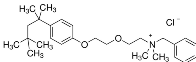
Fig. 1 - Chemical structures of benzethonium chloride. / Structura chimică a clorurii de benzetoniu.
