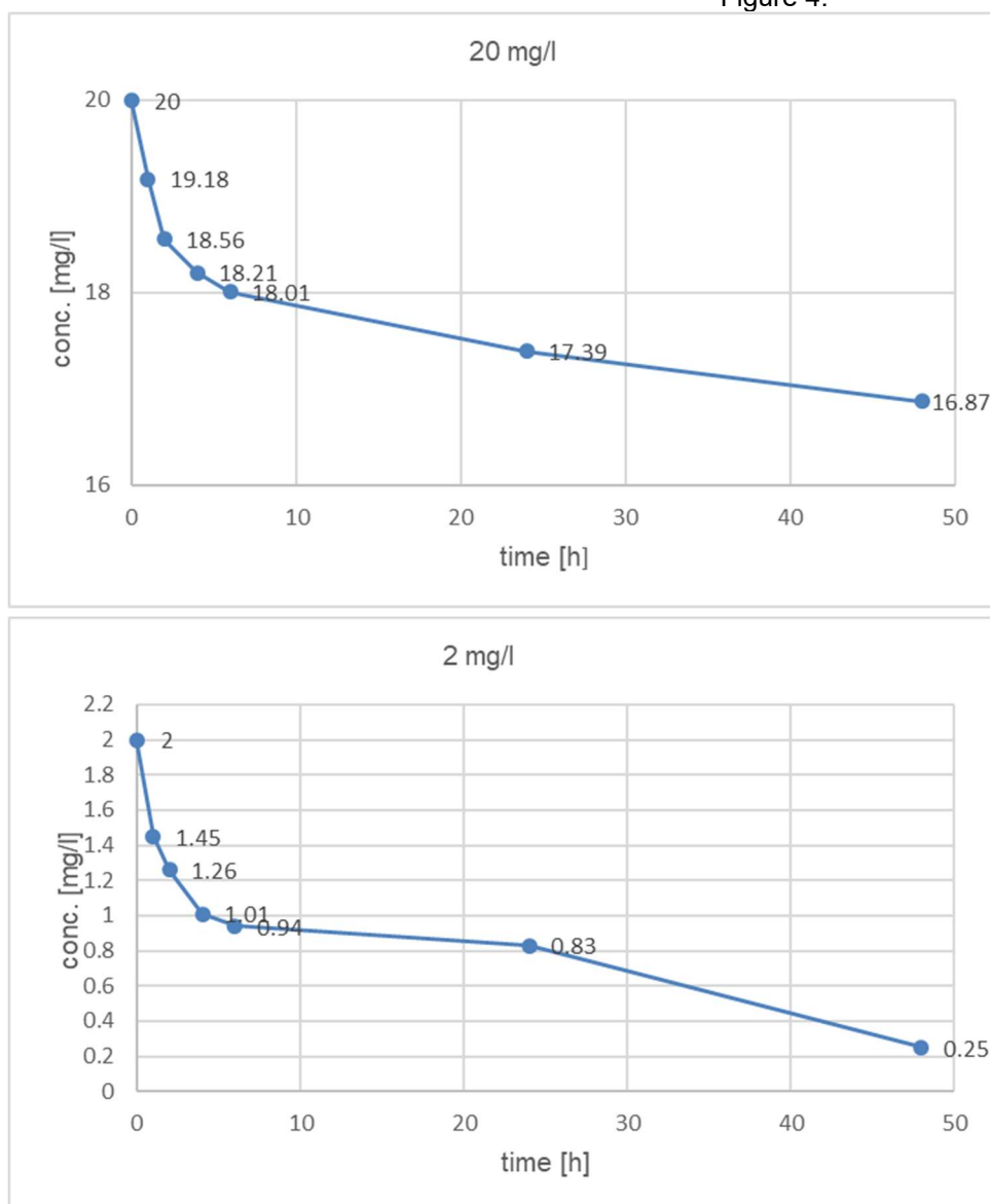
Fig. 4 - Variation of concentration of benzethonium chloride (20 mg/L and 2 mg/L) versus time (h)/ Variația concentrației de clorură de benzetoniu (20 mg/L and 2 mg/L) versus timp (ore).
