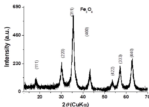
Fig. 2 - XRD patterns of Fe_3O_4 nanomaterial / Difrakția de raze X a nanomaterialului Fe_3O_4 .
